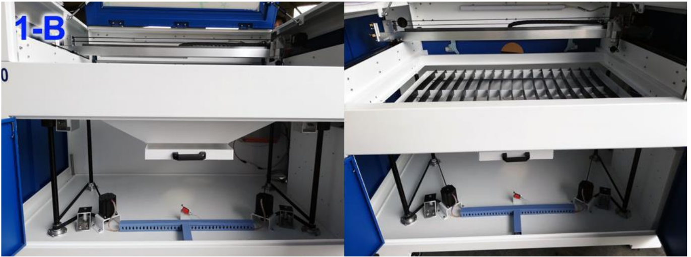
Forgató egység CO2 géphez tokmánnal 2-A tip. / Rotary device for CO2 machine with clamps
