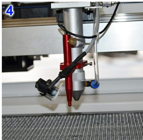
Vörösfényű jelölő és autó fókuszt a lézerfejnél / Red pointer and auto focusing (opció)
